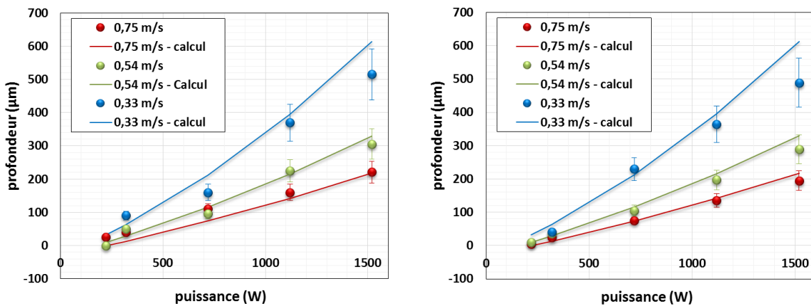
Figure III. 42 : Calcul analytique ( m \approx 5 et n \approx 5 ) des profondeurs fondues sur banc instrumenté (D200) en (a) fusion pleine tôle et (b) avec 60 µm de poudre.
