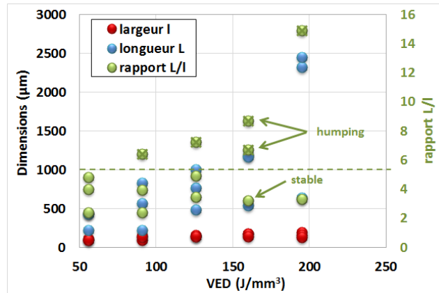
Figure III. 34 : Rapport L/l du bain liquide en fonction du VED (D100_E50).
