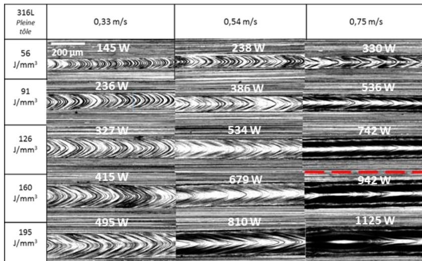
Figure III. 25 : Cartographie des morphologies de cordon pleine tôle pour D100.
