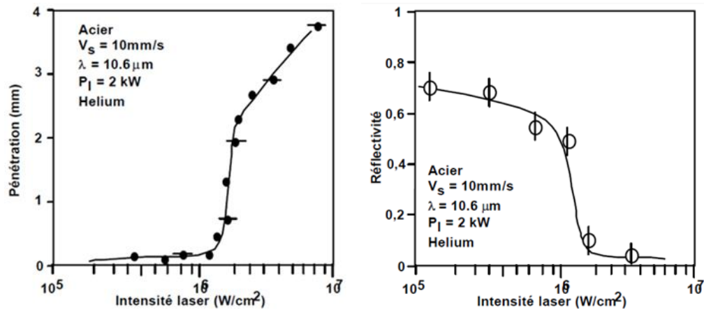
Figure I. 22 : Transition conduction - keyhole sur acier avec un laser \text{CO}_2 . Evolution de la pénétration des cordons de soudage et de la réflectivité du matériau en fonction de l'intensité laser (Fabbro, 2010).
