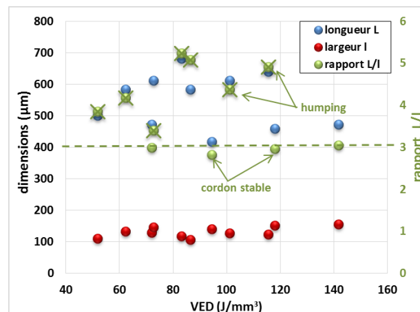
Figure III. 36 : Rapport L/l en fonction du VED pour la machine SLM (D70_E30).
