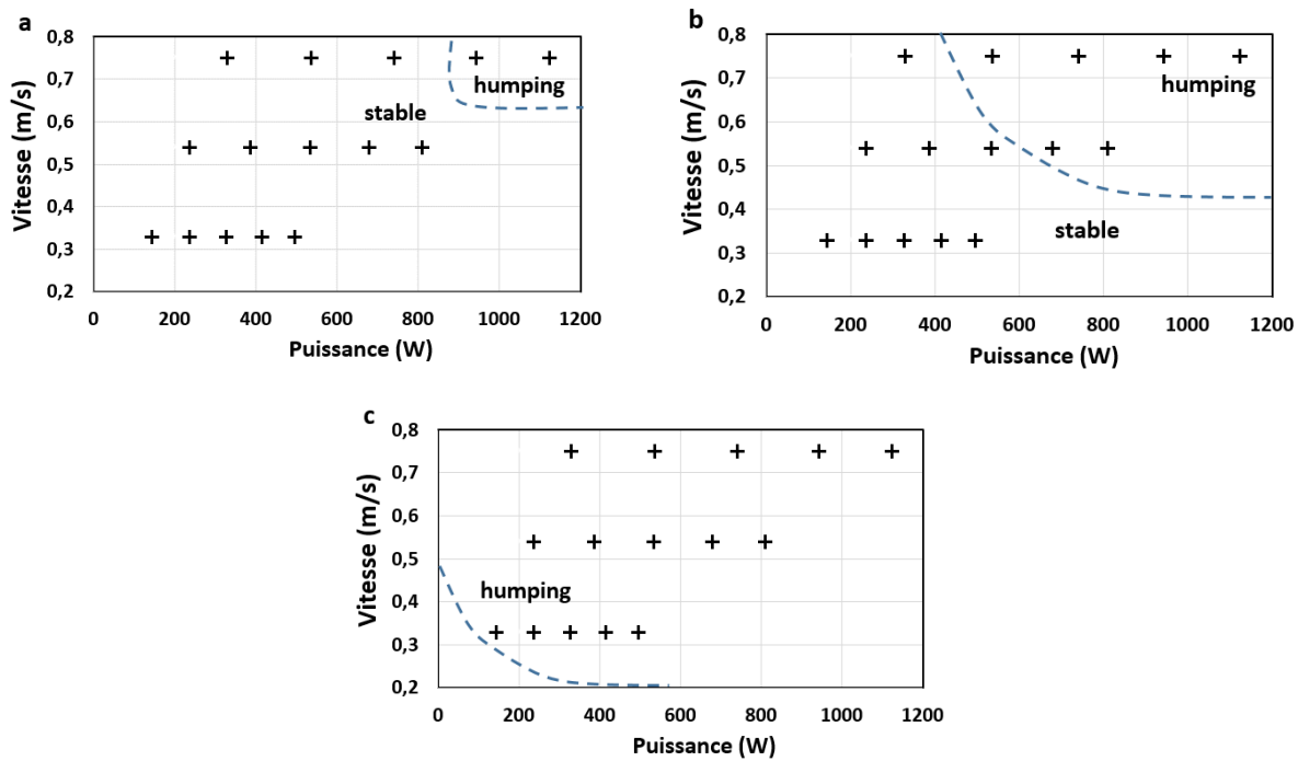
Figure III. 27 : Influence de l'épaisseur de poudre sur les seuils de formation des instabilités (D100) (a) pleine tôle, (b) 50 \mu\text{m} , (c) 100 \mu\text{m} .
