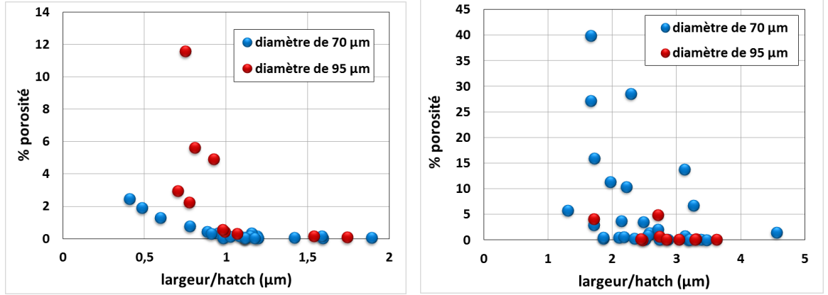
Figure IV. 31 : Taux de porosité en fonction de l/H pour (a) \Delta h = 30 \mu\text{m} , (b) \Delta h = 100 \mu\text{m} .
