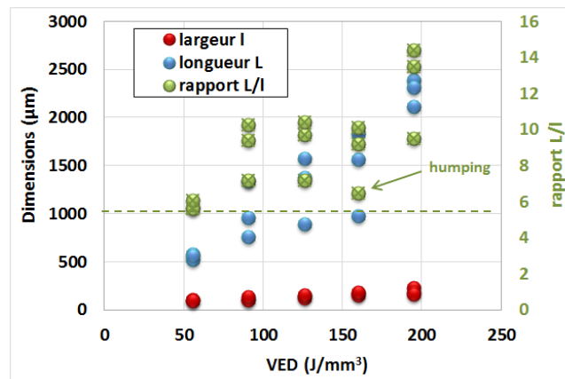
Figure III. 35 : Rapport L/l du bain liquide en fonction du VED (D100_E100).
