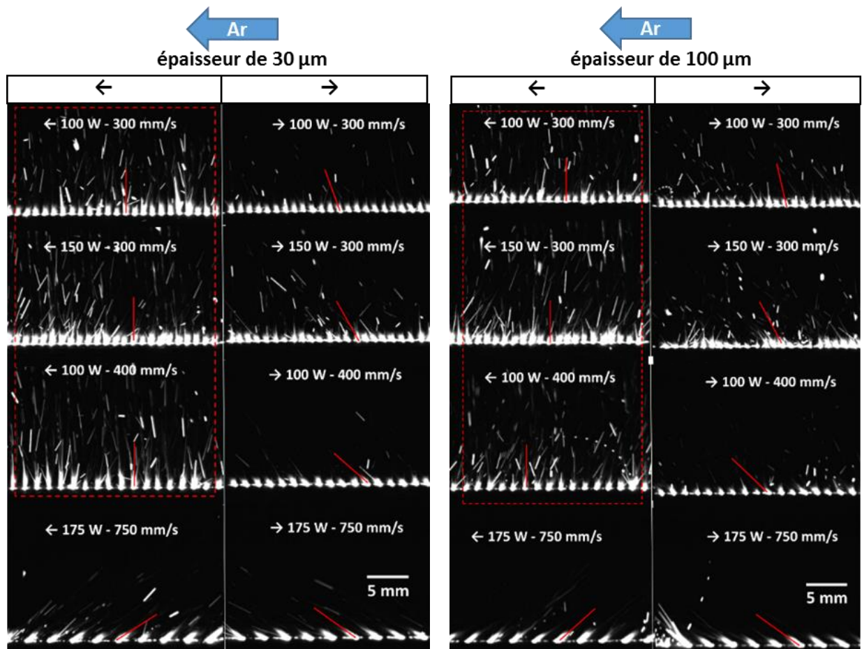
Figure III. 73 : Superposition d'images pour un cordon de 26 mm effectué dans les deux sens de balayage (indiqués par la flèche). Le flux d'argon est dans le sens ← : (a) 30 \mu\text{m} de poudre (b) 100 \mu\text{m} de poudre.
