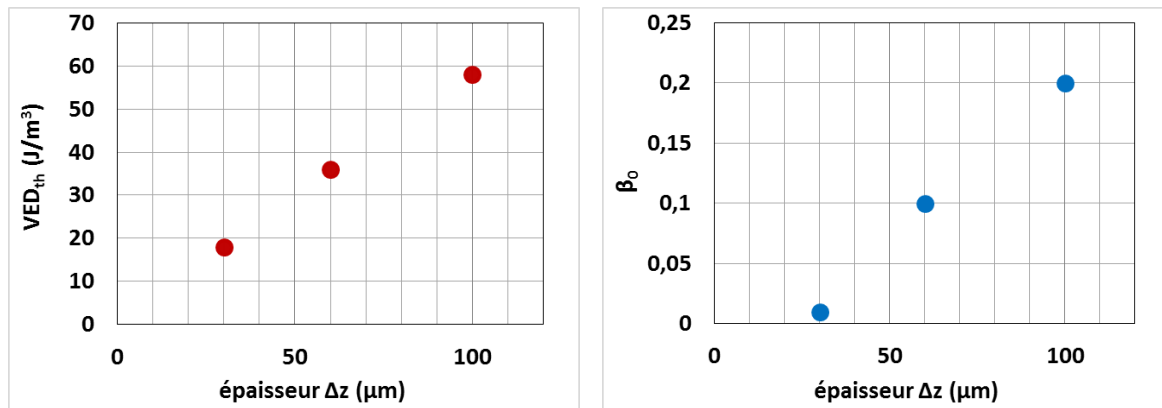
Figure IV. 26 : Fonctions VED_{th} et \beta_0 utilisés dans le modèle.
