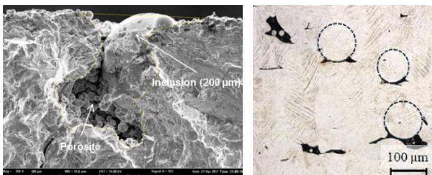
Figure I. 39 : Inclusions et porosités - (a) Rupture en fatigue amorcée sur une porosité à proximité d'une inclusion de grande taille (200 µm) issue des éjections de matière (Ben Haj Khaled, 2017) (b) Pores non sphériques formés à proximité d'inclusions (Kasperovich, 2016).
